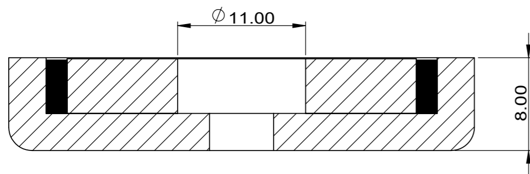
SECTION A-A SCALE 3 : 1
