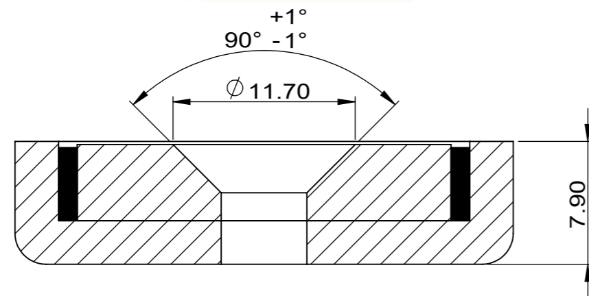
SECTION A-A SCALE 3 : 1
